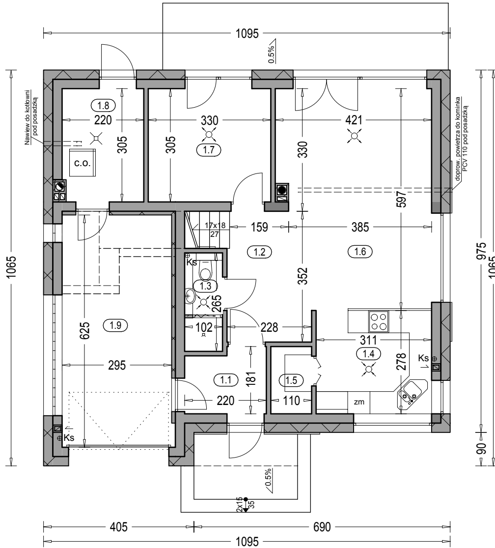
Zestawienie powierzchni parteru
