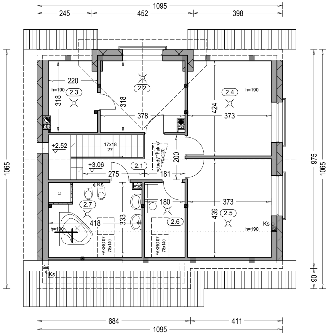
Zestawienie powierzchni poddasza
