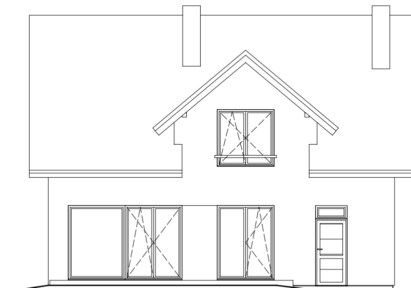
ELEWACJA OGRODOWA
